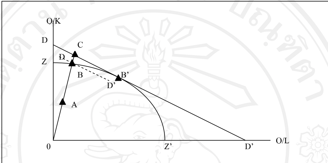
ภาพที่ 2.1 ประสิทธิภาพด้านเทคนิคและการจัดสรรทรัพยากร (Output Oriented Efficiency Measurement)
