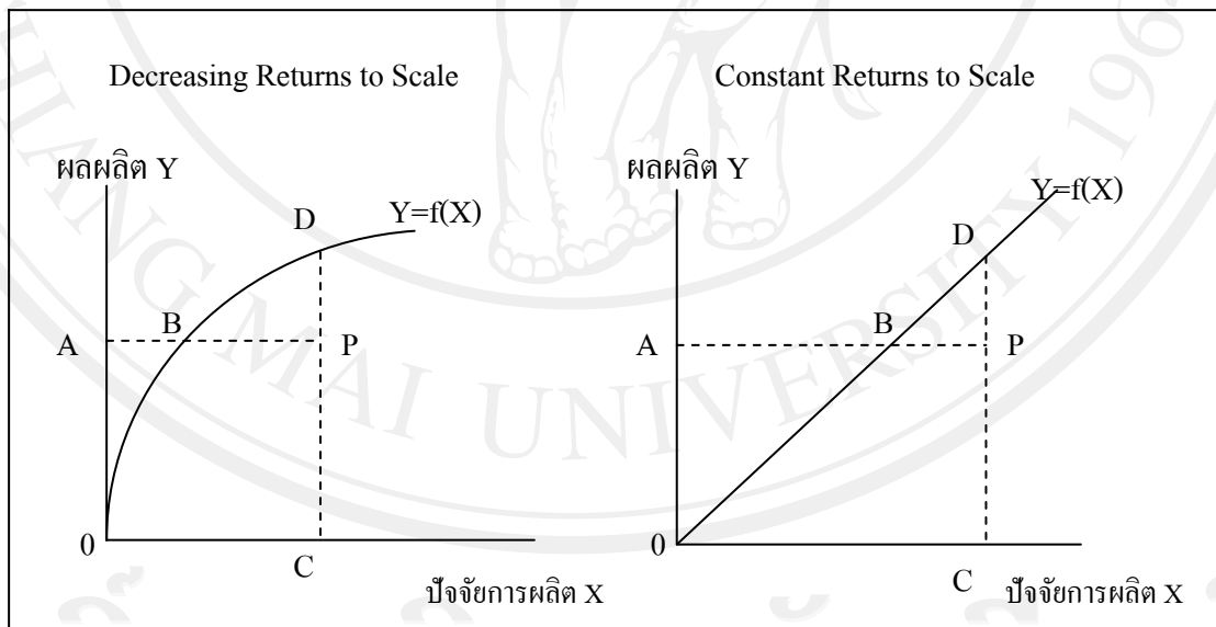
ภาพที่ 2.2 การวัดประสิทธิภาพด้านเทคนิค
