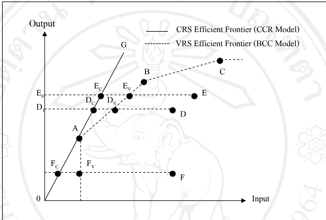
ภาพที่ 2.6 เปรียบเทียบความแตกต่างระหว่างแบบจำลอง CCR และ BCC
