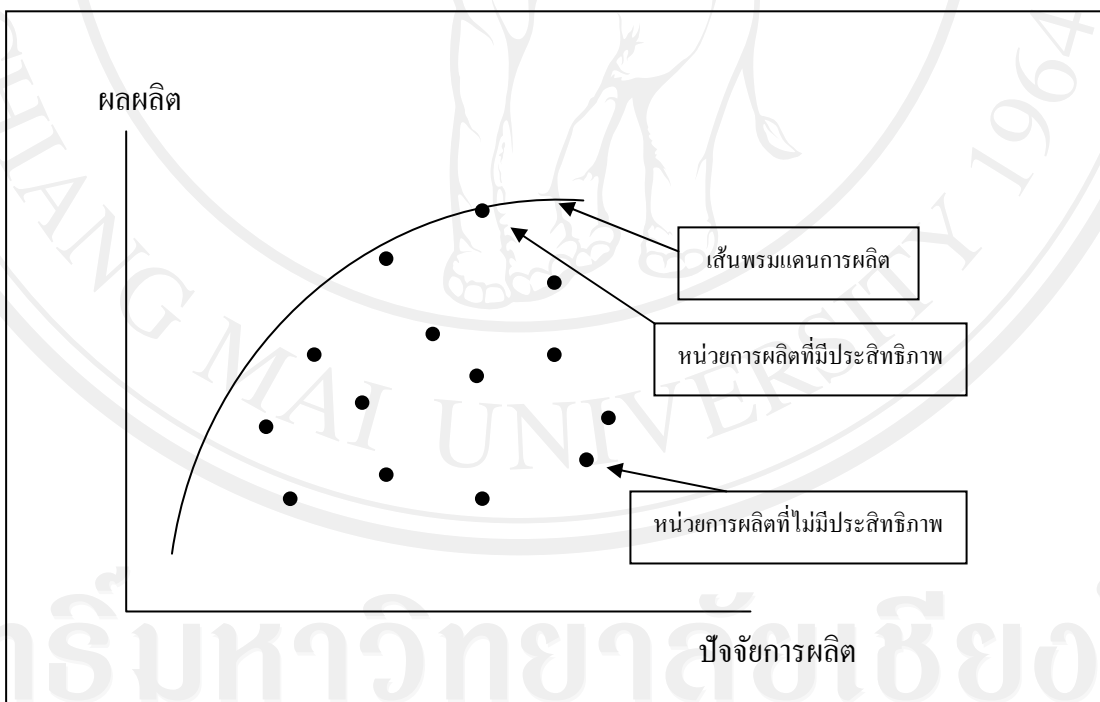
ภาพที่ 2.5 เส้นพรมแดนการผลิตจากการวิเคราะห์เส้นห่อหุ้ม (DEA)
