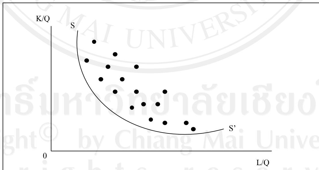
ภาพที่ 2.4 เส้นผลผลิตเท่าที่มีประสิทธิภาพ (Efficient Isoquant)
