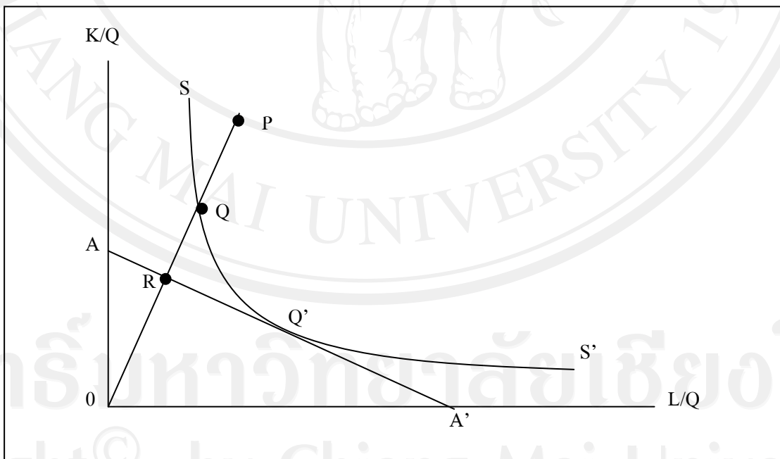
ภาพที่ 2.3 ประสิทธิภาพด้านเทคนิคและการจัดการทรัพยากร (Input Oriented Efficiency Measurement)
