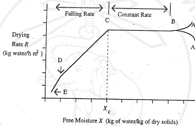
ภาพ 2.5 กราฟอัตราการแห้งสำหรับอาหารชนิดหนึ่งๆ ที่มา : Barbosa-Canovas and Vega-Mercado (1996)
