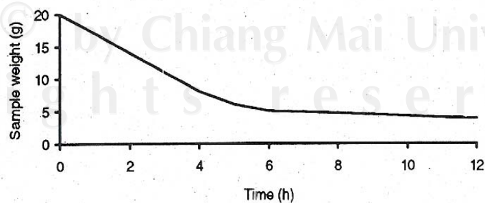
ภาพ 2.3 น้ำหนักที่เปลี่ยนแปลงระหว่างกระบวนการอบแห้ง ที่มา : Barbosa-Canovas and Vega-Mercado (1996)
