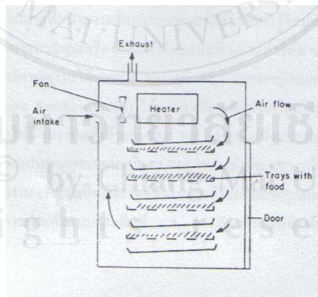
ภาพ 2.7 การทำงานของเครื่องอบแห้งลมร้อนแบบถาดทั่วไป (Karel,1975)
