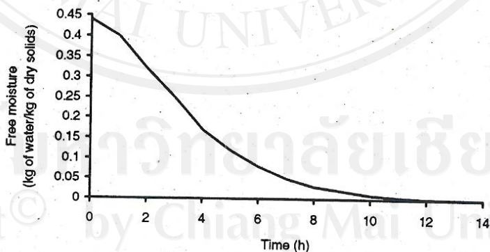
ภาพ 2.4 ปริมาณความชื้นที่เปลี่ยนแปลงตามเวลาการอบแห้ง ที่มา : Barbosa-Canovas and Vega-Mercado (1996)
