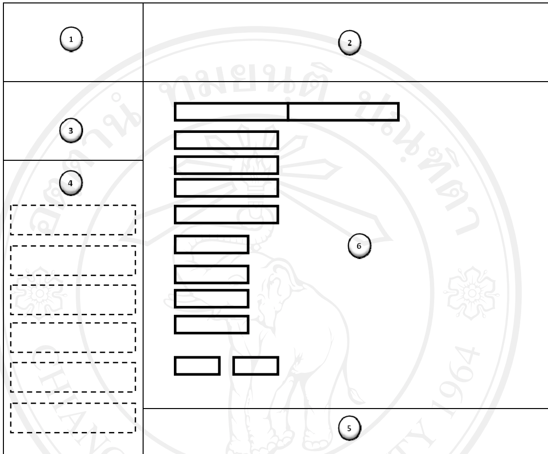
ภาพ 5.16 หน้าจอสำหรับอาจารย์ผู้ประสานรายวิชาในส่วนข้อสอบ
