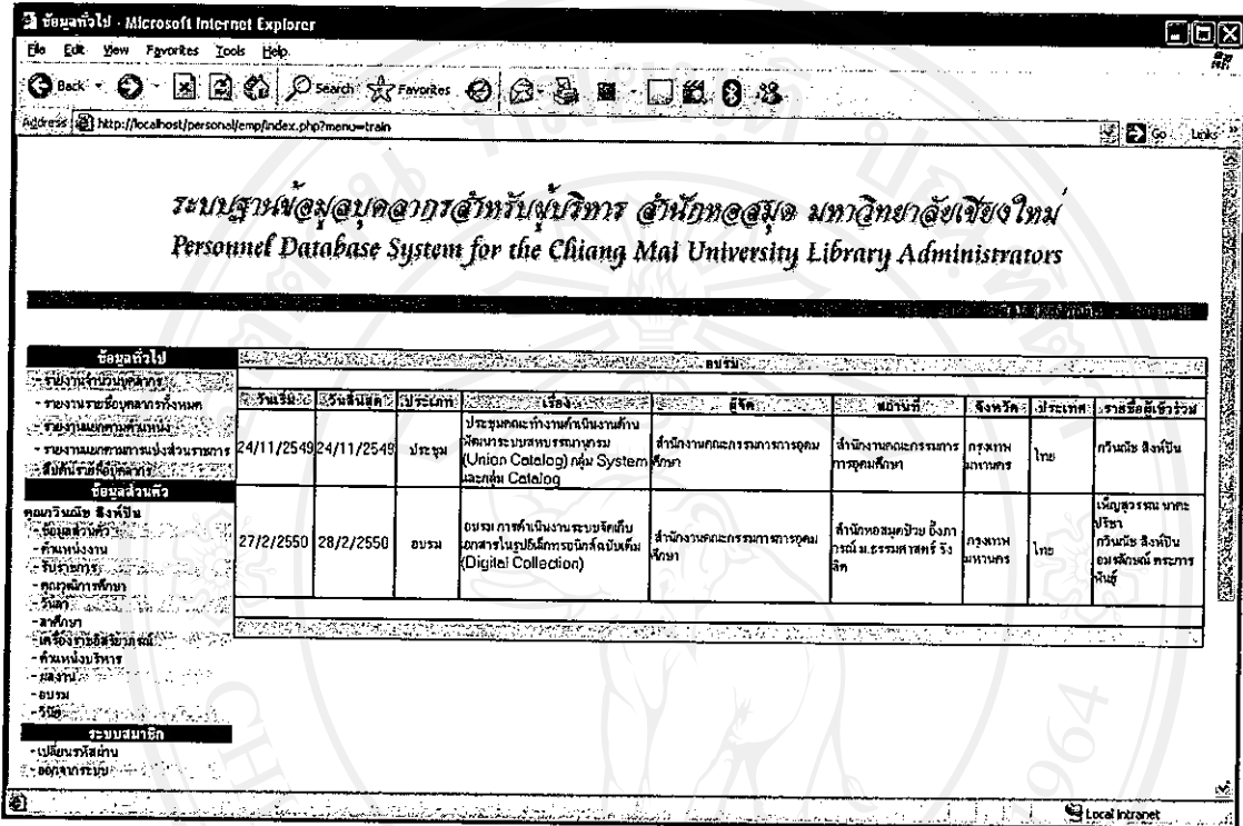
รูป ค.41 หน้าจอแสดงรายละเอียดประวัติการฝึกอบรม / ประชุม / สัมมนา / ดูงาน / ฟังบรรยาย
