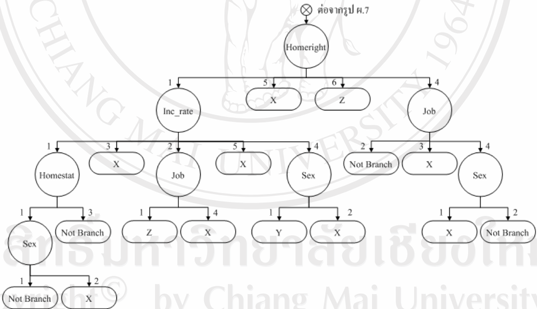
รูป ๗.8 รูปต้นไม้ตัดสินใจโดยใช้ปัจจัย Homeright เมื่อ Loan_rate=4, Hometype=1, Age=3 และ Status=2
