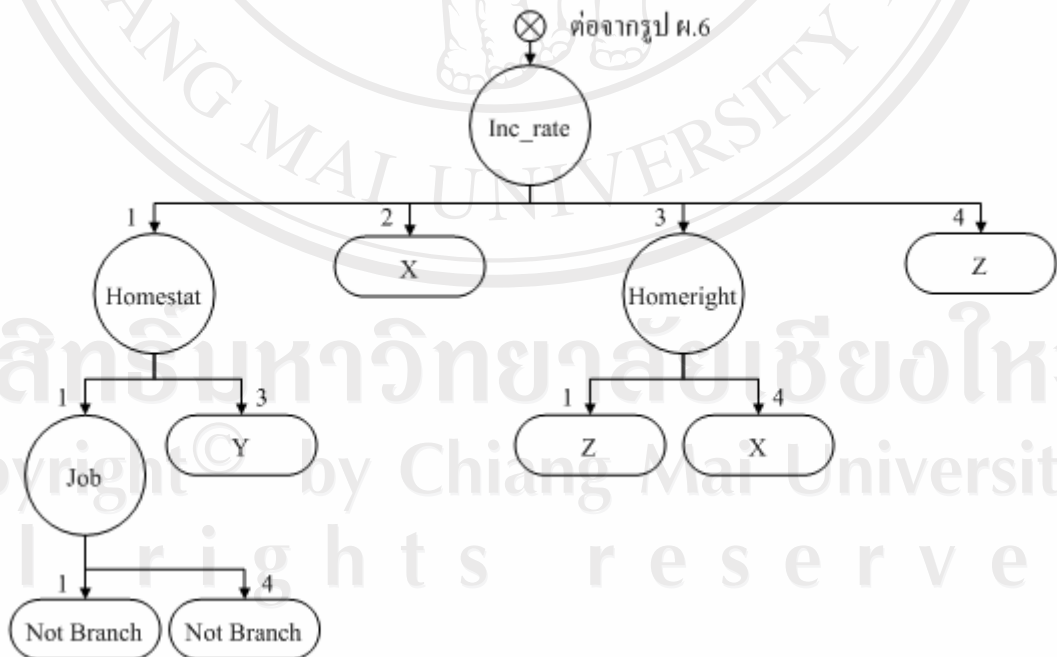
รูป ผ.10 รูปต้นไม้ตัดสินใจโดยใช้ปัจจัย Inc_rate เมื่อ Loan_rate=4, Hometype=1 และ Age=5
