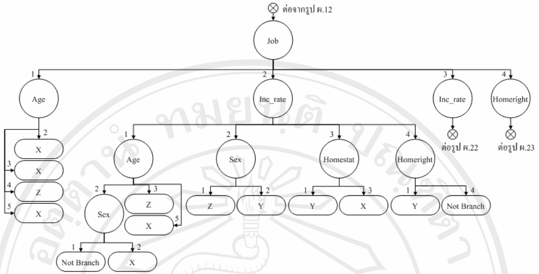
รูป ผ.21 รูปต้นไม้ตัดสินใจโดยใช้ปัจจัย Job เมื่อ Loan_rate=5, Hometype=1 และ Status=6
