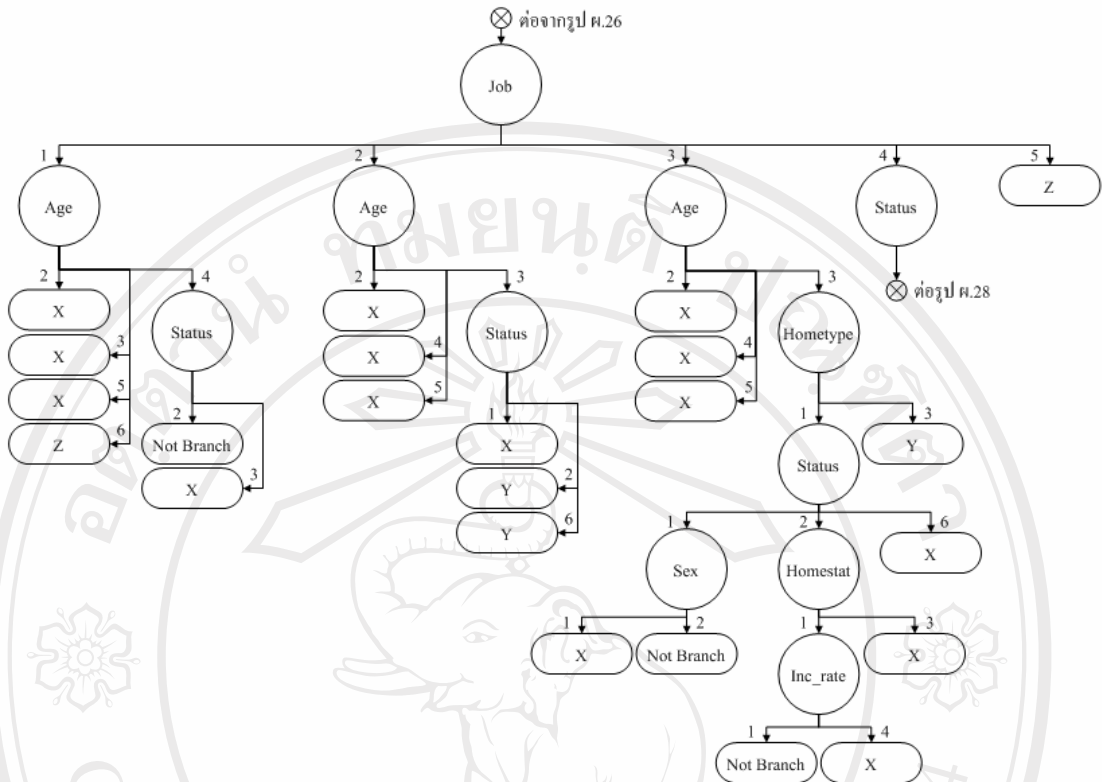
รูป ผ.27 รูปต้นไม้ตัดสินใจโดยใช้ปัจจัย Job เมื่อ Loan_rate=6 และ Homeright=1
