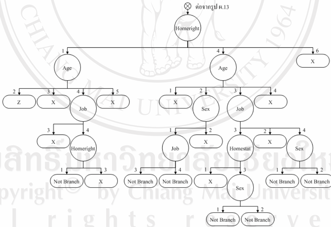
รูป ผ.14 รูปต้นไม้ตัดสินใจโดยใช้ปัจจัย Homeright เมื่อ Loan_rate=5, Hometype=1, Status=1 และ Inc_rate=1
