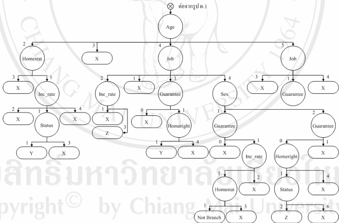
รูป ผ.2 รูปต้นไม้ตัดสินใจโดยใช้ปัจจัย Age เมื่อ Loan_rate=1
