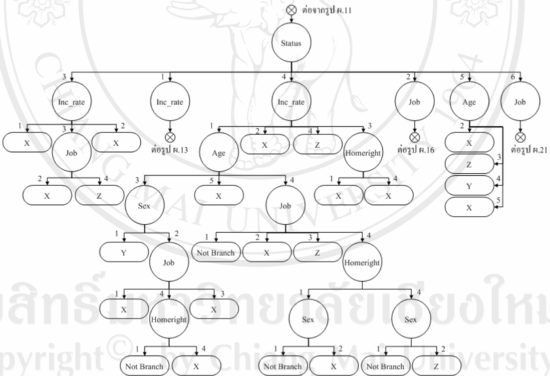
รูป ผ.12 รูปต้นไม้ตัดสินใจโดยใช้ปัจจัย Status เมื่อ Loan_rate=5 และ Hometype=1
