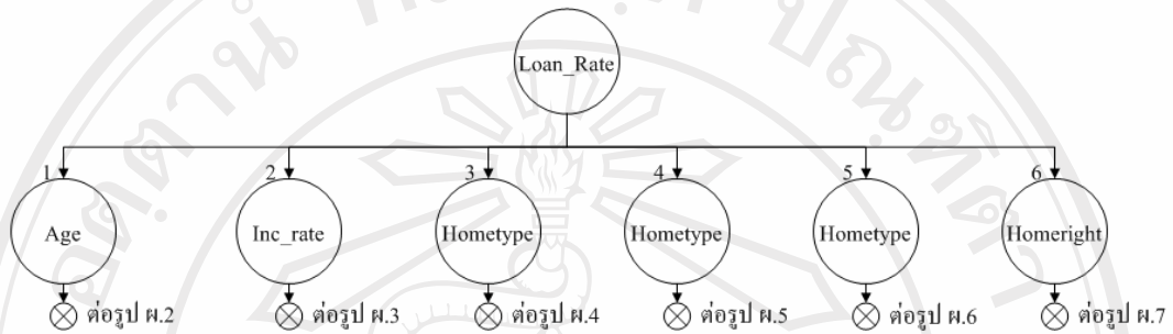
รูป ผ.1 รูปต้นไม้ตัดสินใจโดยใช้ปัจจัย Loan_rate
