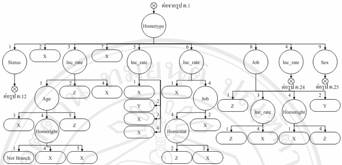
รูป ผ.11 รูปต้นไม้ตัดสินใจโดยใช้ปัจจัย Hometype เมื่อ Loan_rate=5
