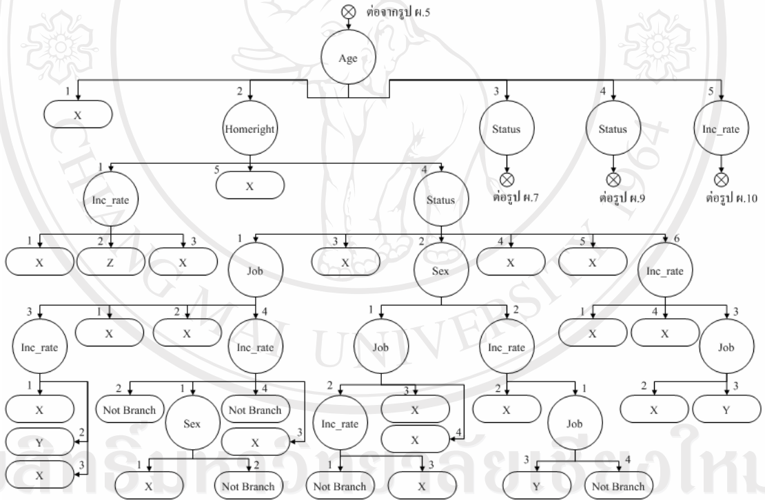
รูป ผ.6 รูปต้นไม้ตัดสินใจโดยใช้ปัจจัย Age เมื่อ Loan_rate=4 และ Hometype=1
