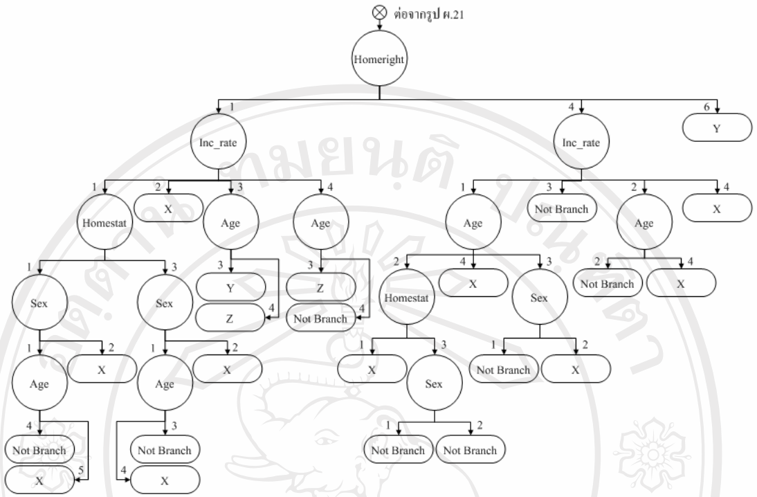
รูป ผ.23 รูปต้นไม้ตัดสินใจโดยใช้ปัจจัย Homeright เมื่อ Loan_rate=5, Hometype=1, Status=6 และ Job=4
