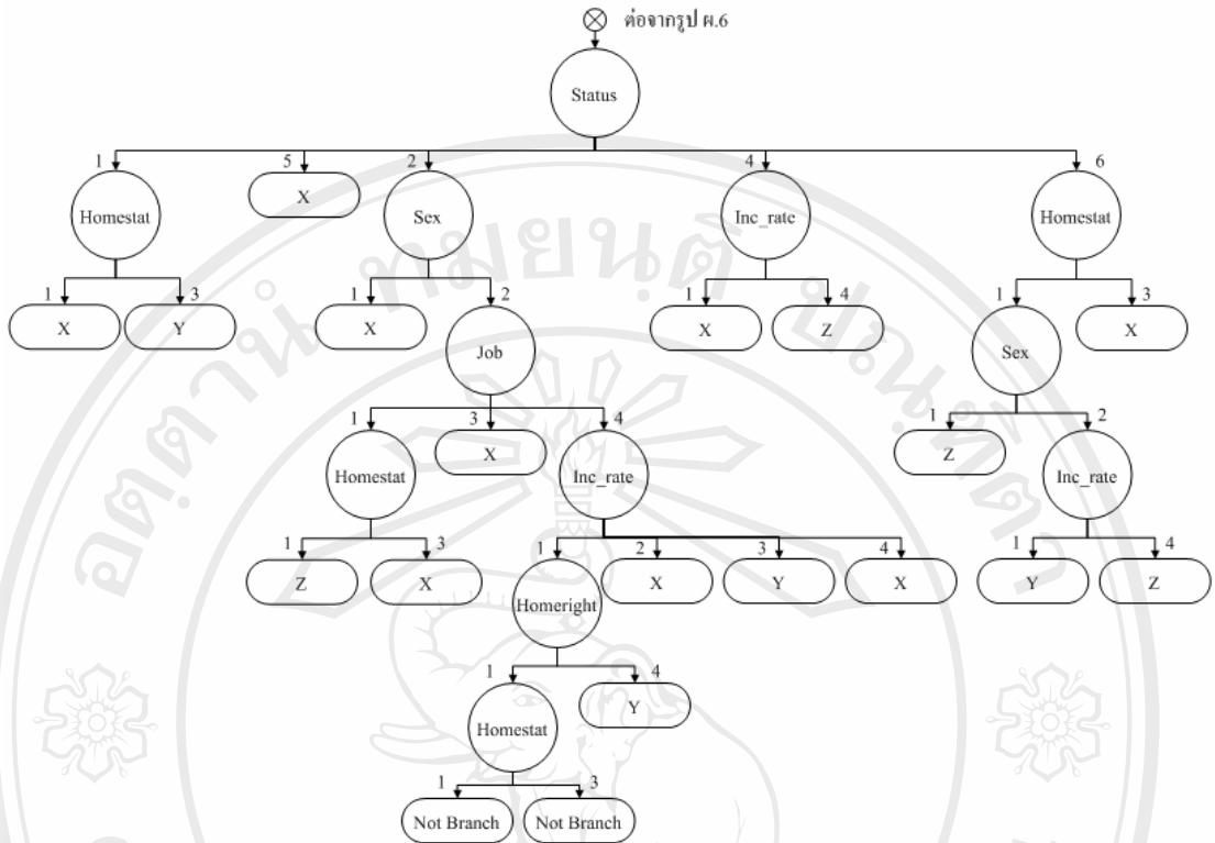
รูป ผ.9 รูปต้นไม้ตัดสินใจโดยใช้ปัจจัย Status เมื่อ Loan_rate=4, Hometype=1 และ Age=4
