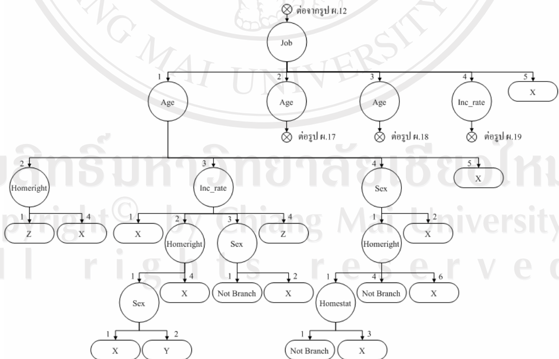
รูป ผ.16 รูปต้นไม้ตัดสินใจโดยใช้ปัจจัย Job เมื่อ Loan_rate=5, Hometype=1 และ Status=2
