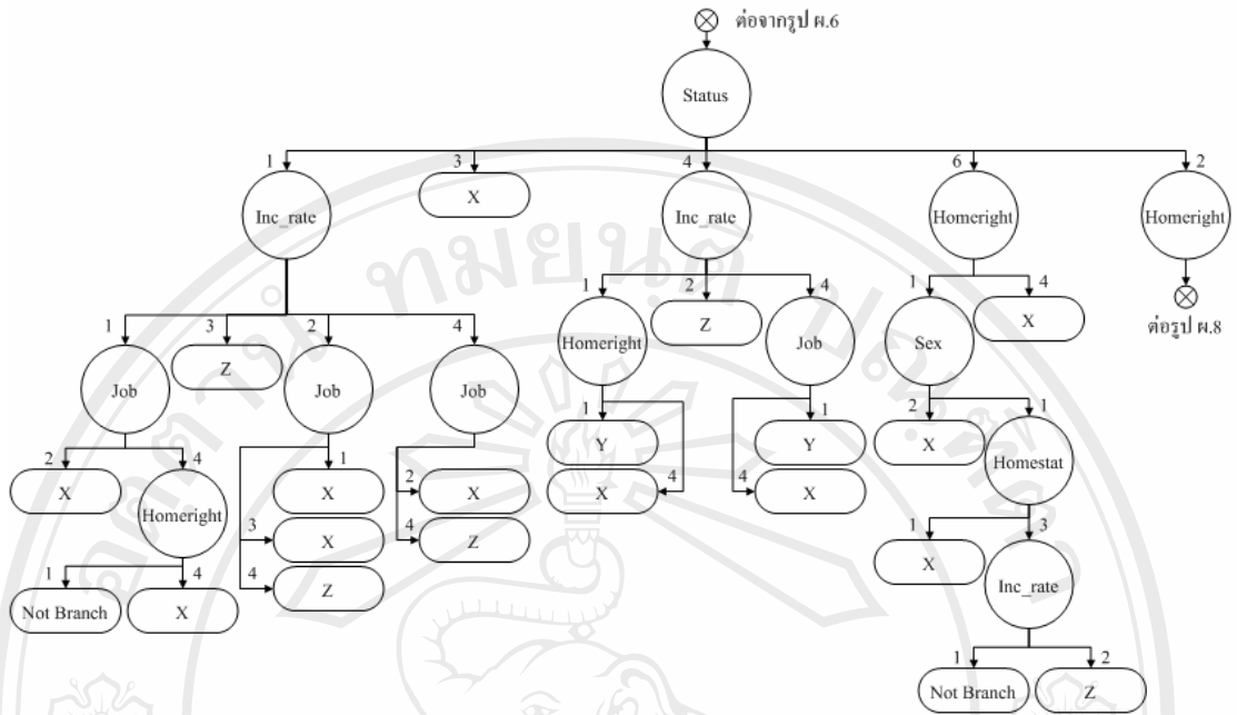
รูป ๗.7 รูปต้นไม้ตัดสินใจโดยใช้ปัจจัย Status เมื่อ Loan_rate=4, Hometype=1 และ Age=3
