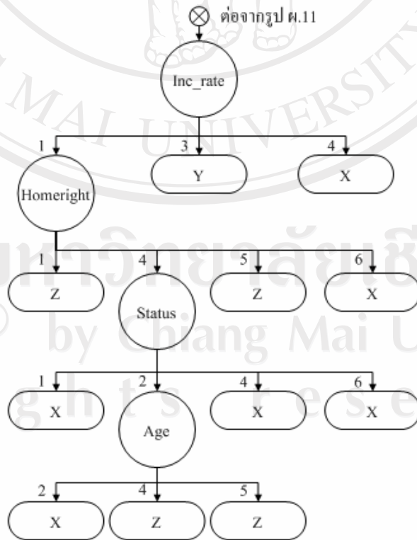
รูป ผ.24 รูปต้นไม้ตัดสินใจโดยใช้ปัจจัย Inc_rate เมื่อ Loan_rate=5 และ Hometype=4
