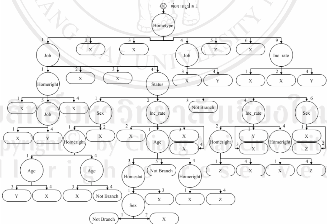
รูป ผ.4 รูปต้นไม้ตัดสินใจโดยใช้ปัจจัย Hometype เมื่อ Loan_rate=3
