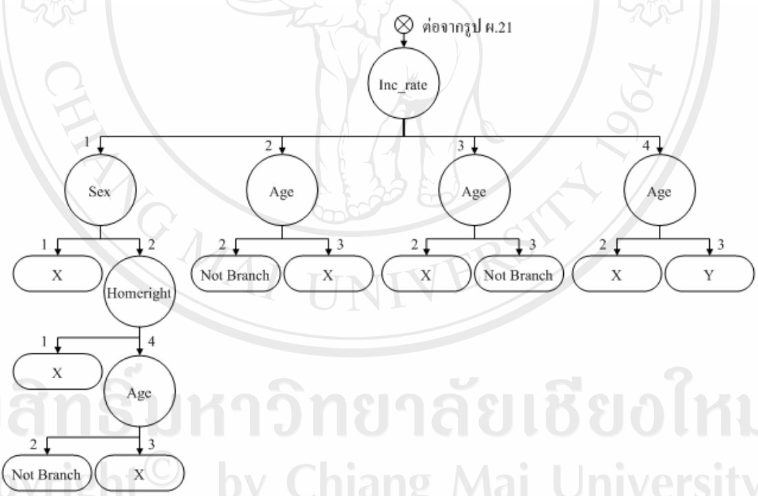
รูป ผ.22 รูปต้นไม้ตัดสินใจโดยใช้ปัจจัย Inc_rate เมื่อ Loan_rate=5, Hometype=1, Status=6 และ Job=3
