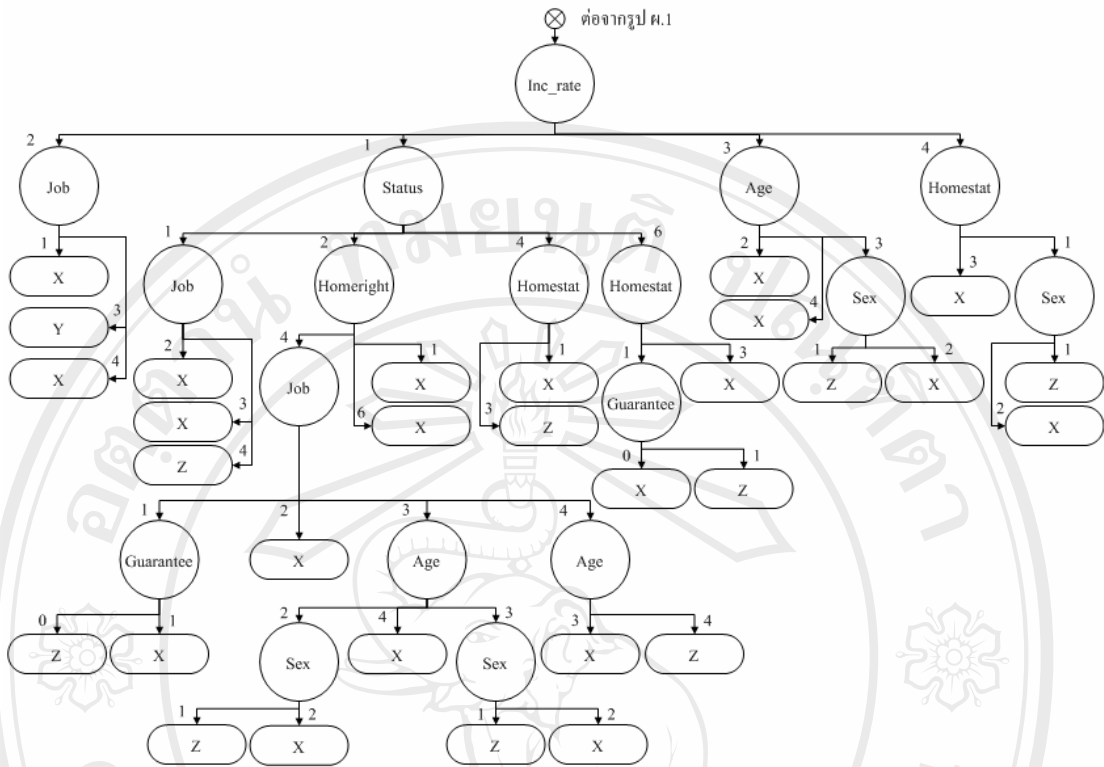
รูป ผ.3 รูปต้นไม้ตัดสินใจโดยใช้ปัจจัย Inc_rate เมื่อ Loan_rate=2
