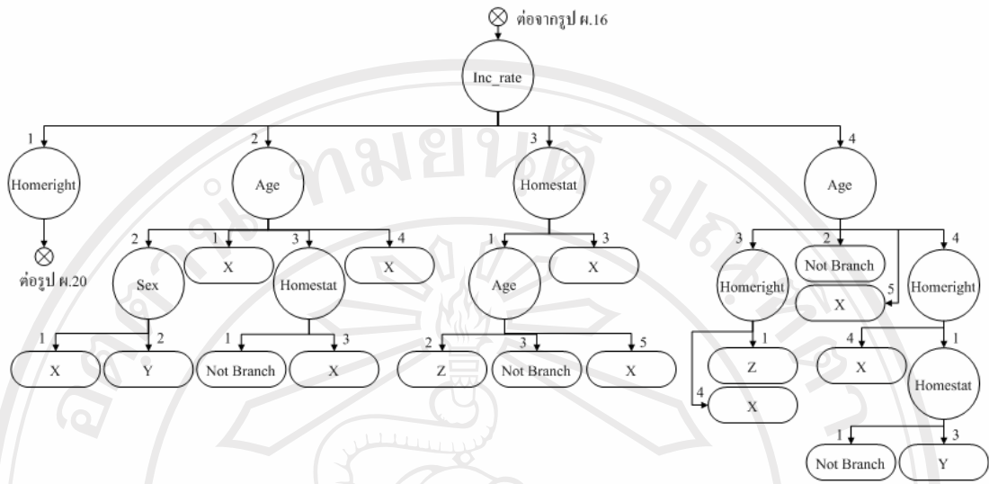
รูป ผ.19 รูปต้นไม้ตัดสินใจโดยใช้ปัจจัย Inc_rate เมื่อ Loan_rate=5, Hometype=1, Status=2 และ Job=4
