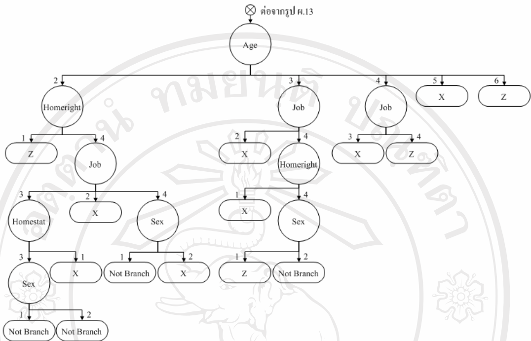
รูป ผ.15 รูปต้นไม้ตัดสินใจโดยใช้ปัจจัย Age เมื่อ Loan_rate=5, Hometype=1, Status=1 และ Inc_rate=3
