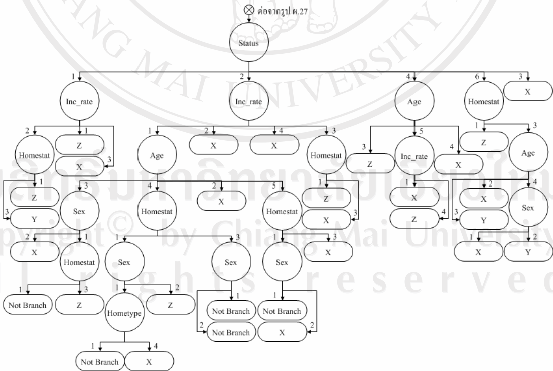
รูป ผ.28 รูปต้นไม้ตัดสินใจโดยใช้ปัจจัย Status เมื่อ Loan_rate=6, Homeright=1 และ Job=4
