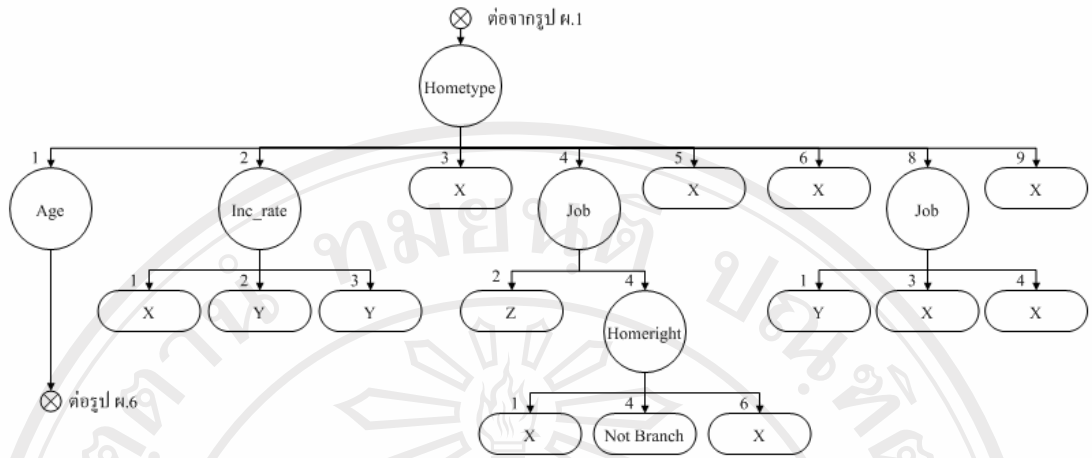
รูป ผ.5 รูปต้นไม้ตัดสินใจโดยใช้ปัจจัย Hometype เมื่อ Loan_rate=4
