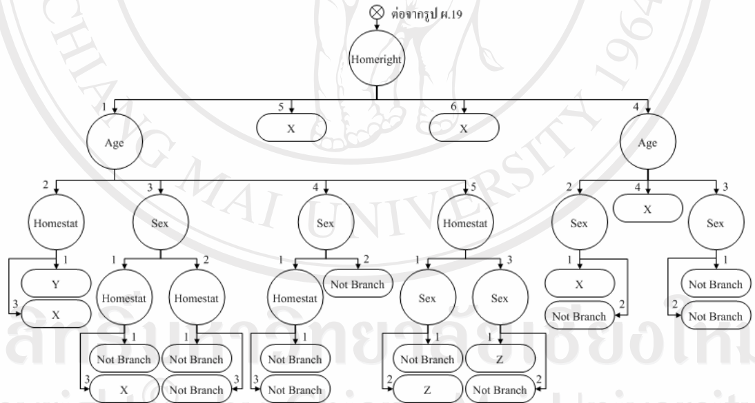
รูป ผ.20 รูปต้นไม้ตัดสินใจโดยใช้ปัจจัย Homeright เมื่อ Loan_rate=5, Hometype=1, Status=2, Job=4 และ Inc_rate=1
