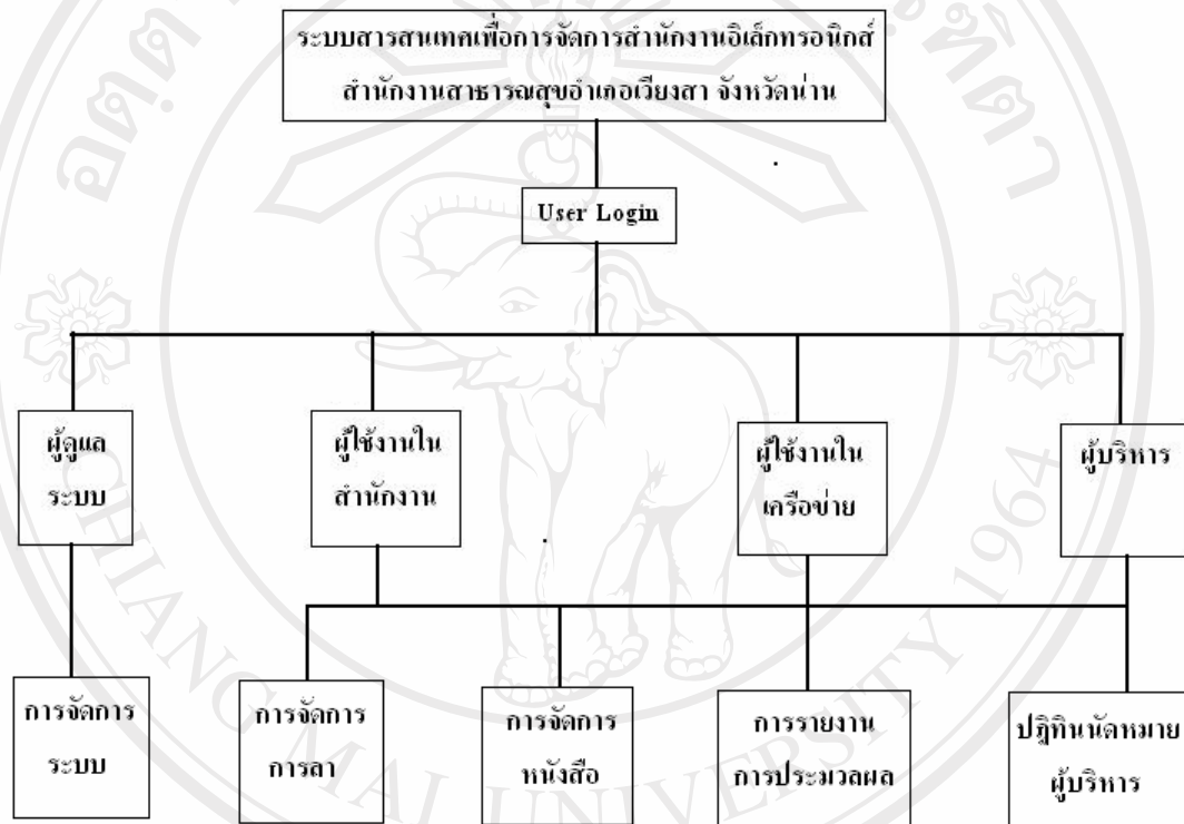
รูป 5.12 แสดงโครงสร้างของเว็บไซต์และการเชื่อมโยงเว็บเพจในเว็บไซต์ของระบบสารสนเทศเพื่อการจัดการสำนักงานอิเล็กทรอนิกส์ สำนักงานสาธารณสุขอำเภอเวียงสา
