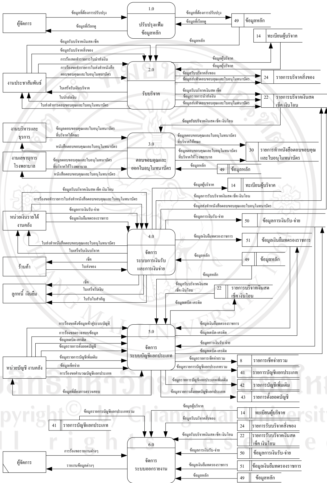
รูป 4.3 แผนผังการไหลของข้อมูลระดับที่ 0 ระบบสารสนเทศเงินบริจาคและกองทุน
