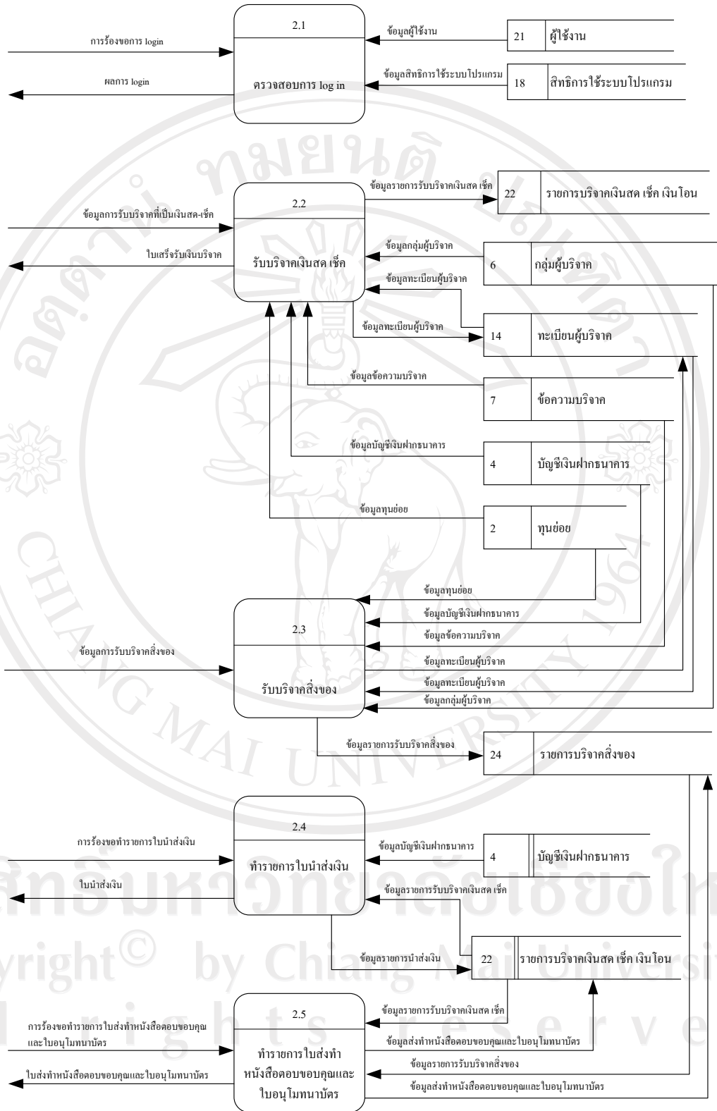
รูป 4.5 แผนผังการไหลของข้อมูลระดับที่ 1 ของบวนการที่ 2.0 รับบริจาค
