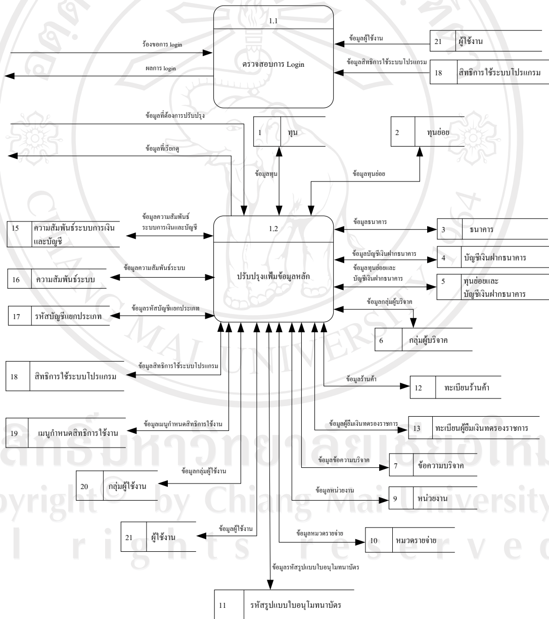
รูป 4.4 แผนผังการไหลของข้อมูลระดับที่ 1 ของ กระบวนการที่ 1.0 ปรับปรุงเพิ่มข้อมูลหลัก
