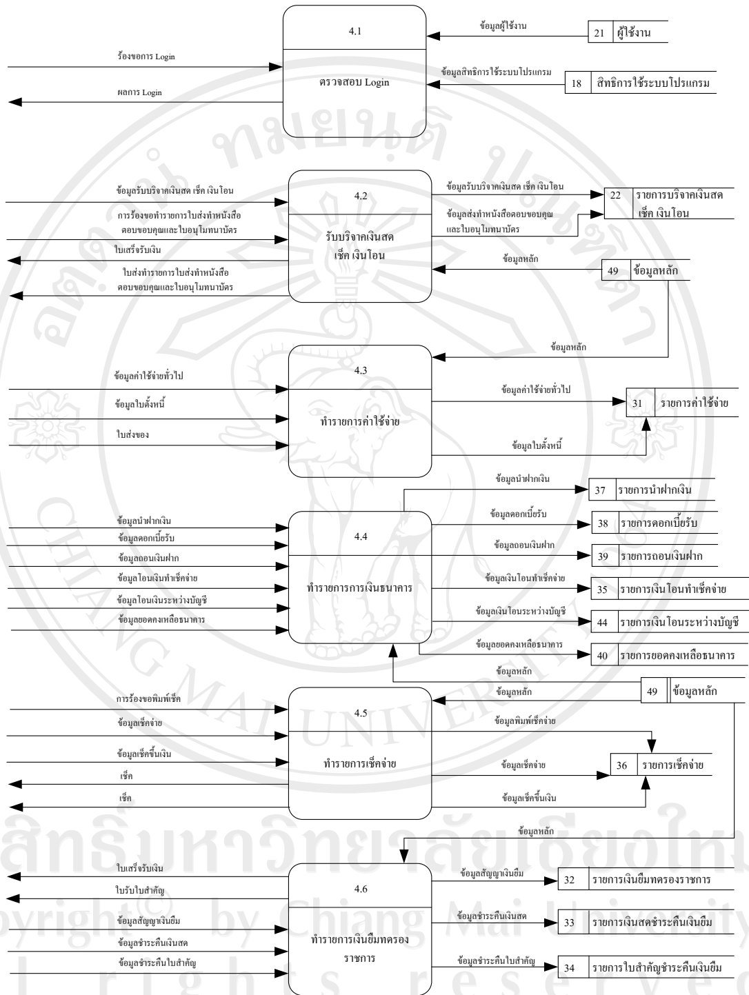
รูป 4.7 แผนผังการไหลของข้อมูลระดับที่ 1 ของกระบวนการที่ 4.0 จัดการระบบการเงินรับและการเงินจ่าย
