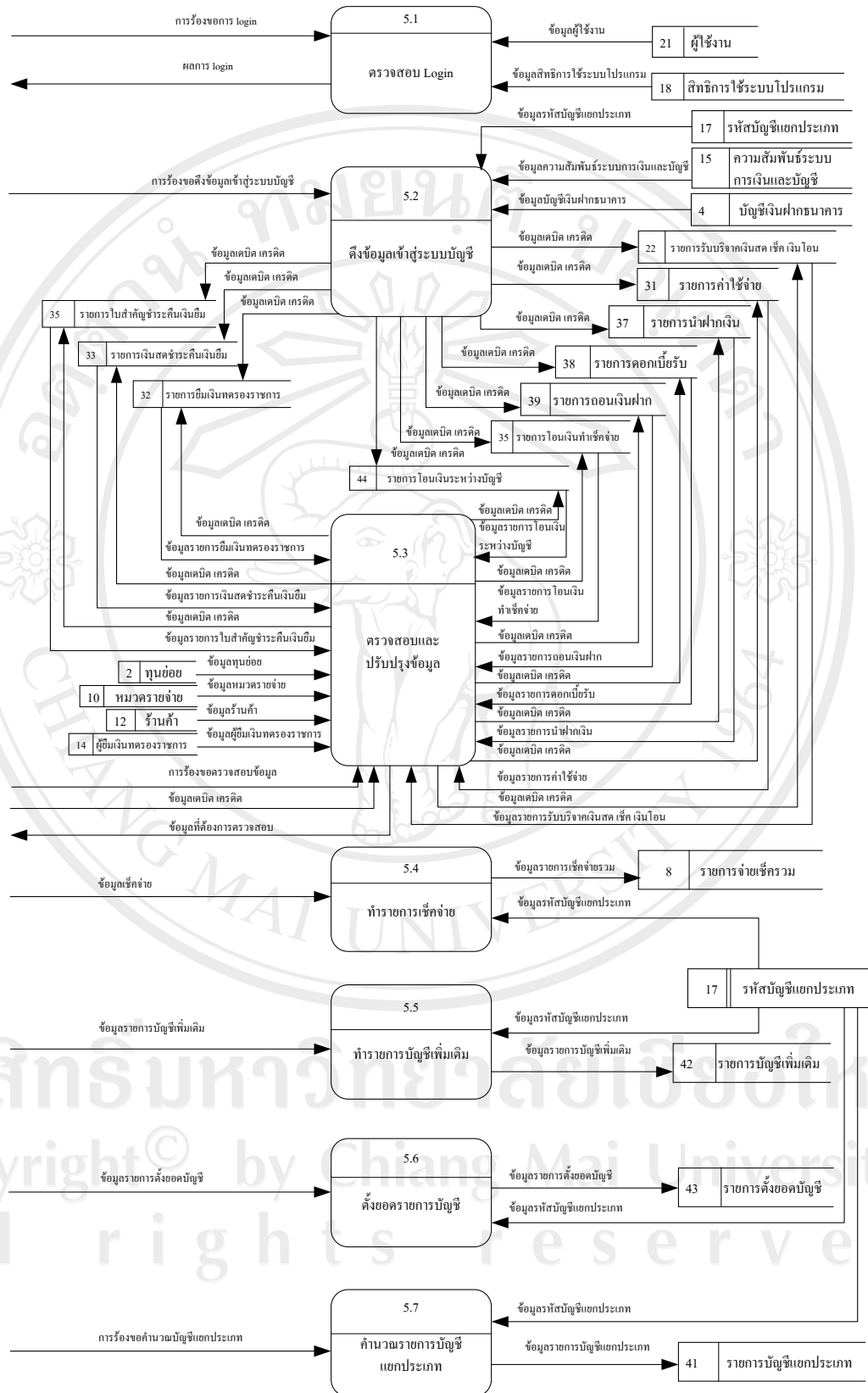
รูป 4.8 แผนผังการไหลของข้อมูลระดับที่ 1 ของกระบวนการที่ 5.0 จัดการระบบบัญชีแยกประเภท
