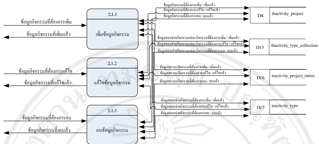
รูป 4.4 แผนผังกระแสข้อมูลระดับที่ 2 กระบวนการ 2.1 จัดการข้อมูลกิจกรรม
