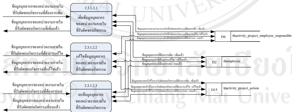
รูป 4.14 แผนผังกระแสข้อมูลระดับที่ 4 กระบวนการ 2.3.1.2 จัดการข้อมูล บุคลากรของหน่วยงานภายในที่รับผิดชอบกิจกรรม
