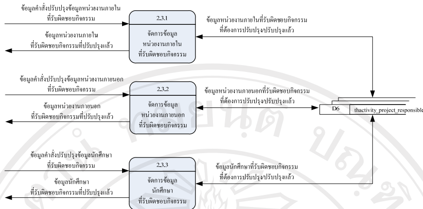
รูป 4.6 แผนผังกระแสข้อมูลระดับที่ 2 กระบวนการ 2.3 จัดการข้อมูลผู้รับผิดชอบกิจกรรม
