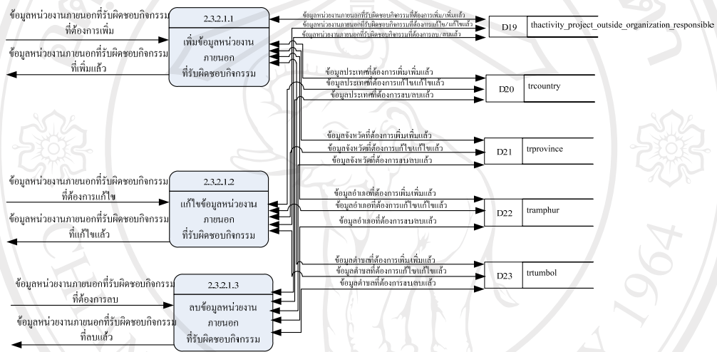
รูป 4.15 แผนผังกระแสข้อมูลระดับที่ 4 กระบวนการ 2.3.2.1 จัดการข้อมูล หน่วยงานภายนอกที่รับผิดชอบกิจกรรม
