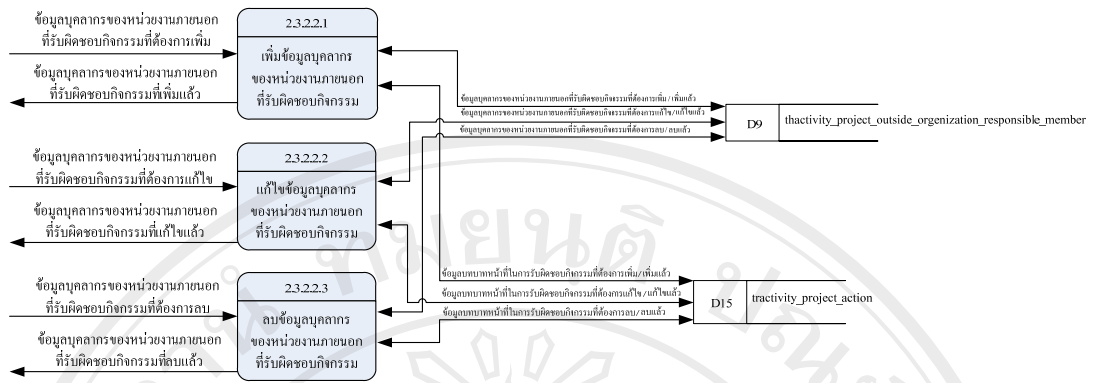
รูป 4.16 แผนผังกระแสข้อมูลระดับที่ 4 กระบวนการ 2.3.2.2 จัดการข้อมูลบุคลากรของหน่วยงานภายนอกที่รับผิดชอบกิจกรรม
