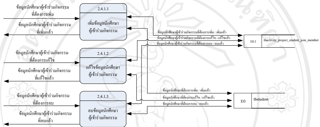
รูป 4.12 แผนผังกระแสข้อมูลระดับที่ 3 กระบวนการ 2.4.1 จัดการข้อมูลรายชื่อนักศึกษาผู้เข้าร่วมกิจกรรม
