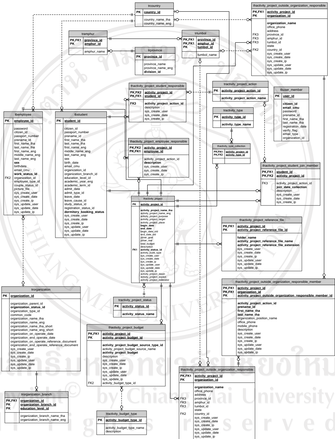
รูป 4.17 แผนภาพแสดงความสัมพันธ์ของระบบฐานข้อมูล
