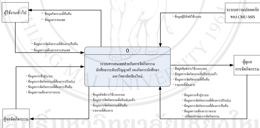
รูป 4.1 แผนผังบริบทของระบบสารสนเทศสำหรับการจัดกิจกรรม นักศึกษาระดับปริญญาตรี กองกิจการนักศึกษา มหาวิทยาลัยเชียงใหม่
