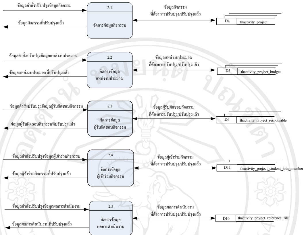
รูป 4.3 แผนผังกระแสข้อมูลระดับที่ 1 กระบวนการ 2.0 จัดการข้อมูล
