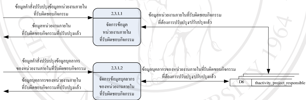
รูป 4.9 แผนผังกระแสข้อมูลระดับที่ 3 กระบวนการ 2.3.1 จัดการข้อมูลหน่วยงานภายในที่รับผิดชอบกิจกรรม
