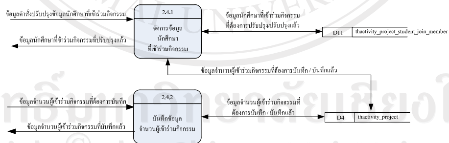
รูป 4.7 แผนผังกระแสข้อมูลระดับที่ 2 กระบวนการ 2.4 จัดการข้อมูลผู้เข้าร่วมกิจกรรม
