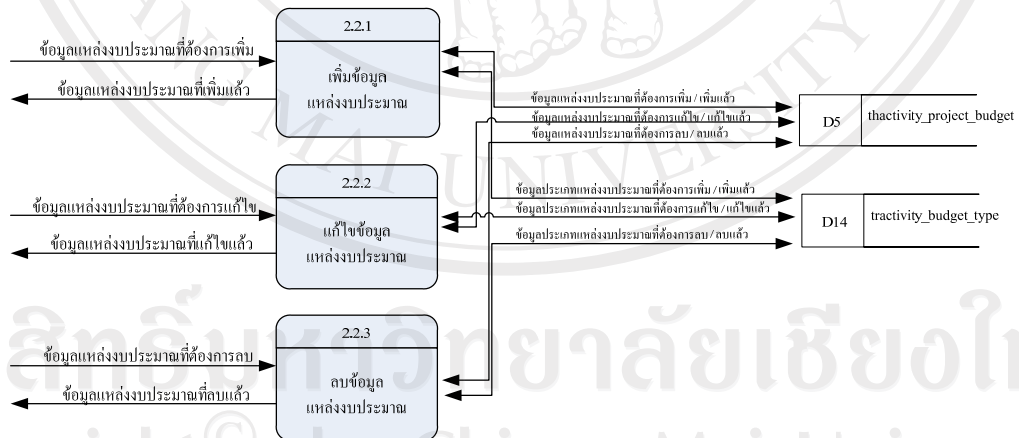
รูป 4.5 แผนผังกระแสข้อมูลระดับที่ 2 กระบวนการ 2.2 จัดการข้อมูลแหล่งงบประมาณ
