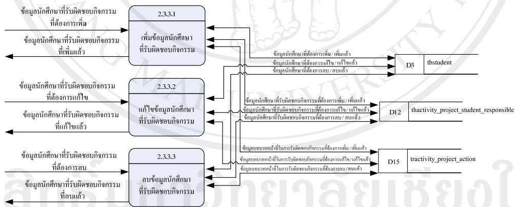
รูป 4.11 แผนผังกระแสข้อมูลระดับที่ 3 กระบวนการ 2.3.3 จัดการข้อมูลนักศึกษาที่รับผิดชอบกิจกรรม
