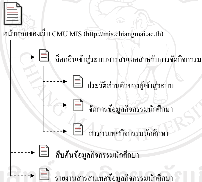
รูป 4.18 การเชื่อมโยงไปยังหน้าจอต่างๆ ในส่วนของระบบ
