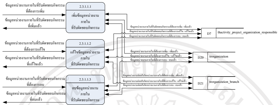
รูป 4.13 แผนผังกระแสข้อมูลระดับที่ 4 กระบวนการ 2.3.1.1 จัดการข้อมูล หน่วยงานภายในที่รับผิดชอบกิจกรรม
