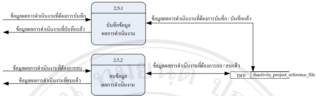
รูป 4.8 แผนผังกระแสข้อมูลระดับที่ 2 กระบวนการ 2.5 จัดการข้อมูลผลการดำเนินงาน
