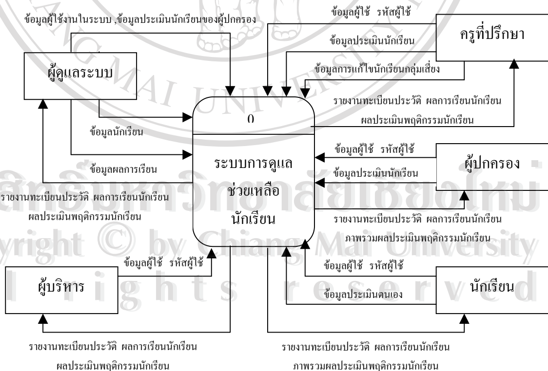
รูป 3.1 แผนภาพบริบท (Context Diagram) ของระบบ
