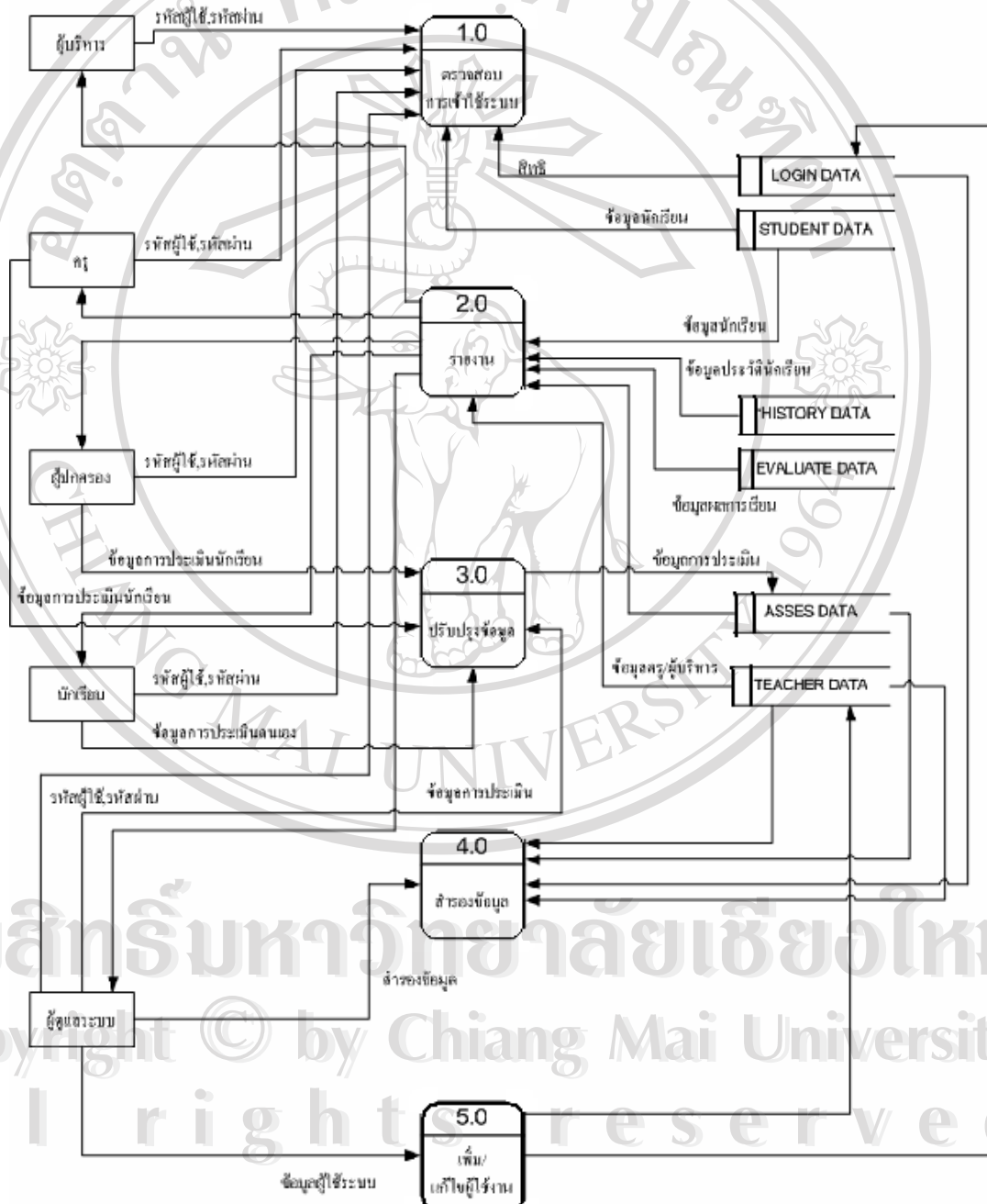
รูป 3.2 แสดงผังการไหลของข้อมูลระดับที่ 0
