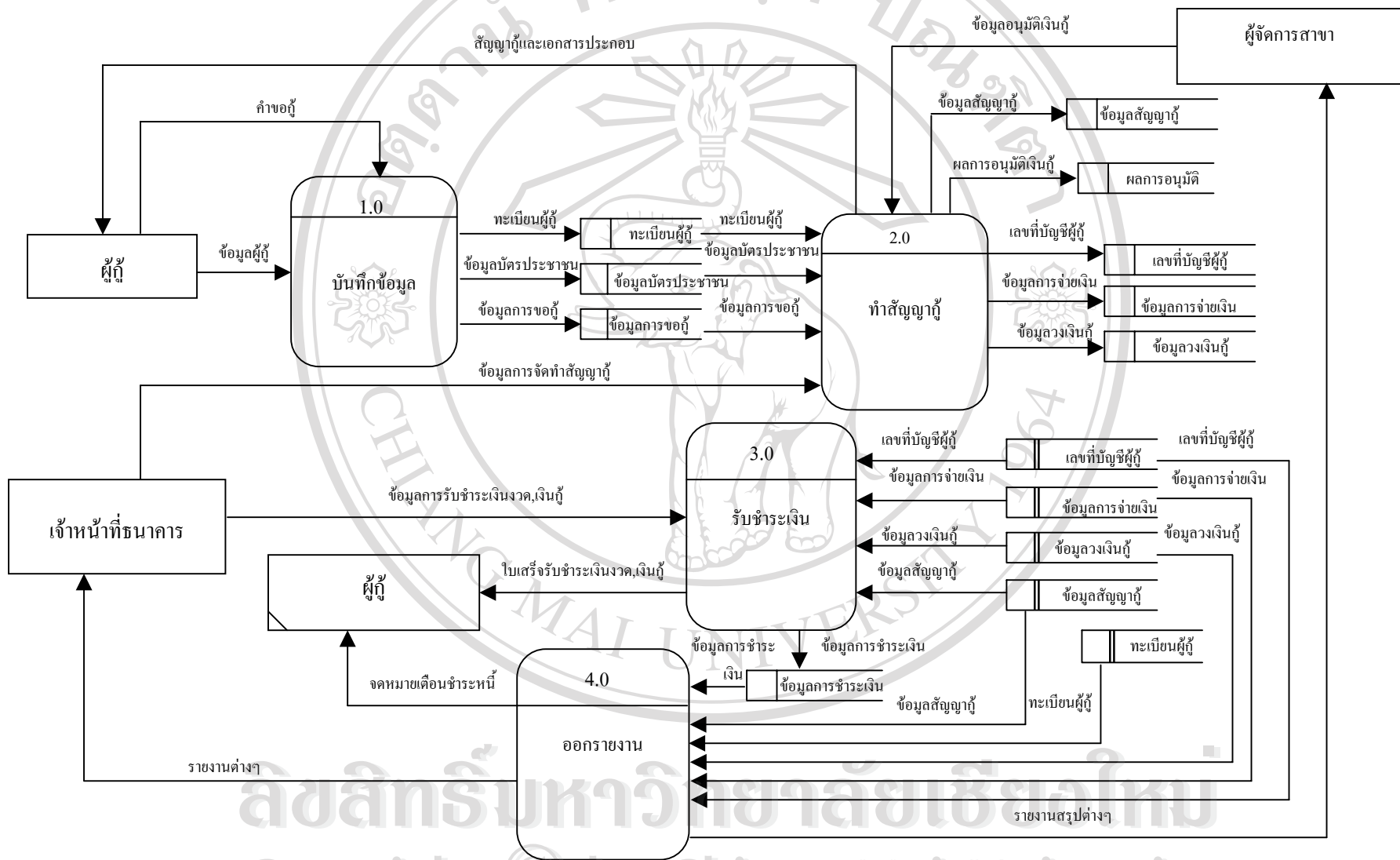
รูป 3.7 Data Flow Diagram(Level 0) ระบบสารสนเทศเพื่อสนับสนุนการจัดการงานดินเชื้อ โครงการธนาคารประชาชน
