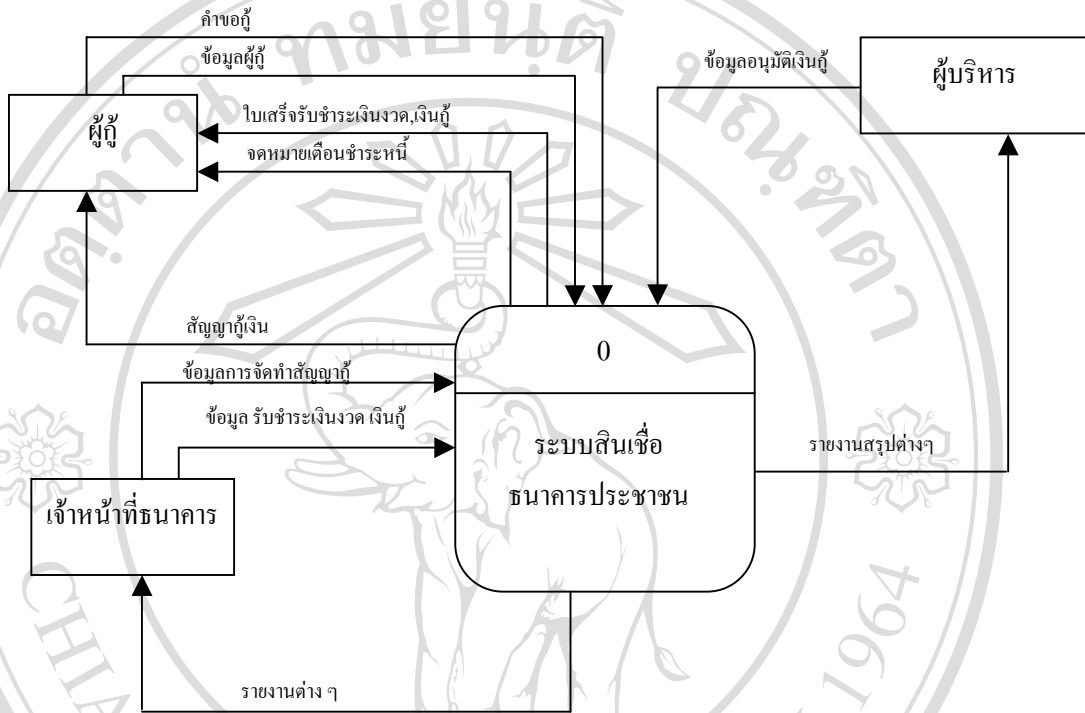
รูป 3.6 Context Diagram ระบบสารสนเทศเพื่อสนับสนุนการจัดการงานสินเชื่อ โครงการธนาคารประชาชน
