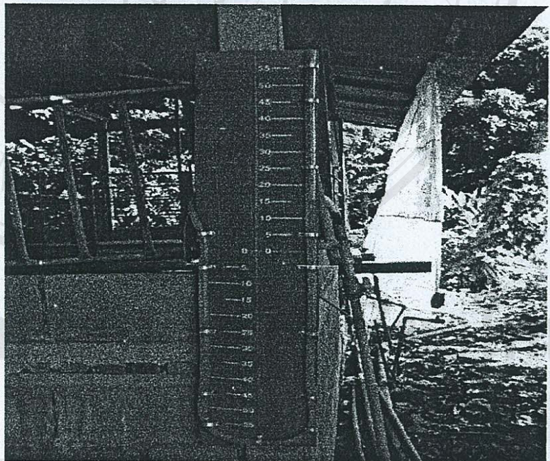
ภาพแสดงระบบวัดแรงดันของก๊าซ และปริมาณของก๊าซที่อยู่ในถังหมัก
