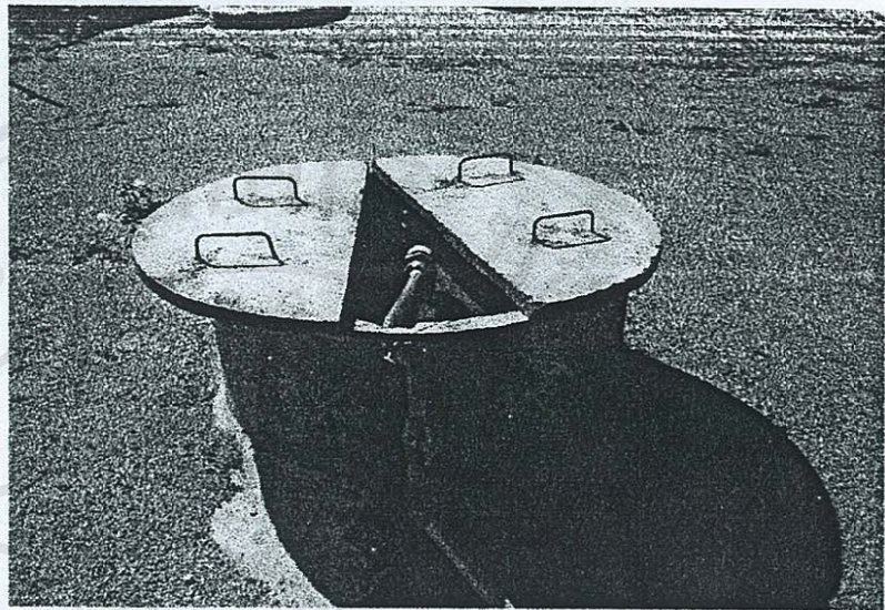
ภาพแสดงการต่อท่อก๊าซชีวภาพออกจากถังหมัก
